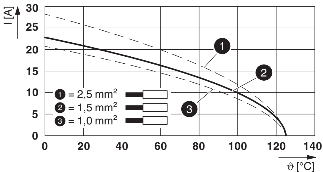
Diagrama derating para conductores rígidos
