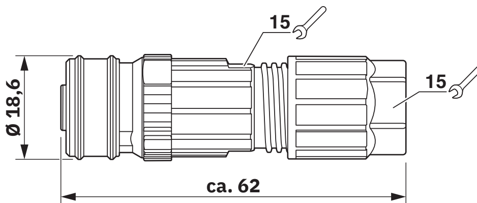
Maßzeichnung
