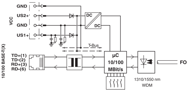
Schéma fonctionnel
