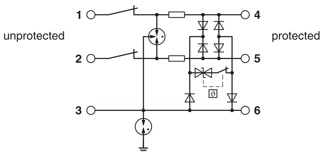
Diagrama eléctrico
