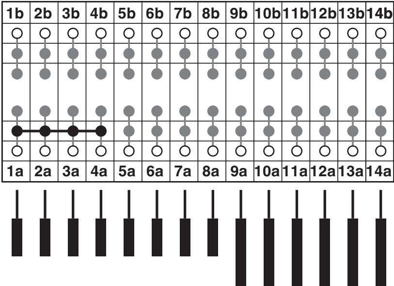
Diagrama eléctrico
