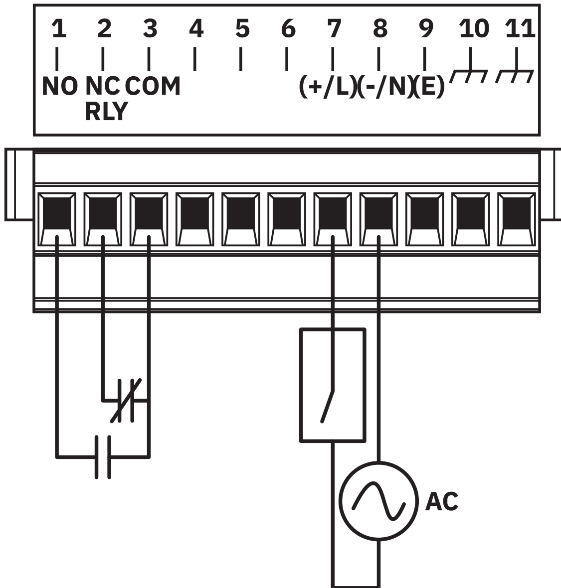
Anschlusszeichnung
