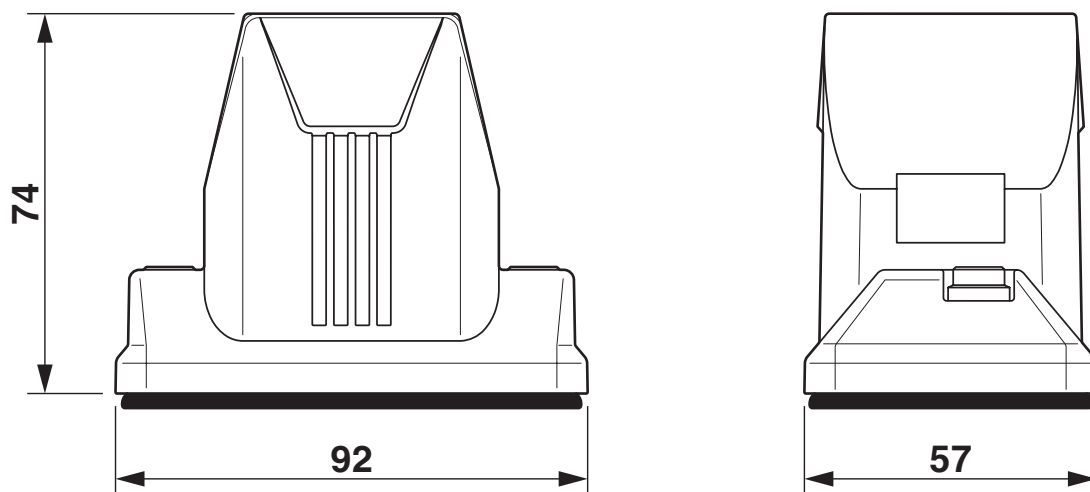
Dessin coté
