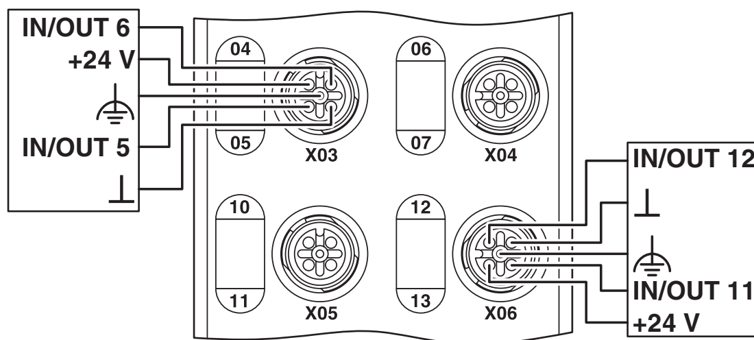
Dibujo de conexión
