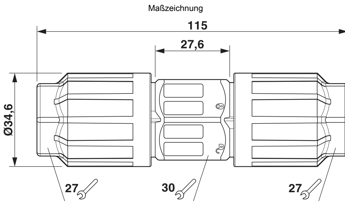
Maßzeichnung QPD C 5x2,5
