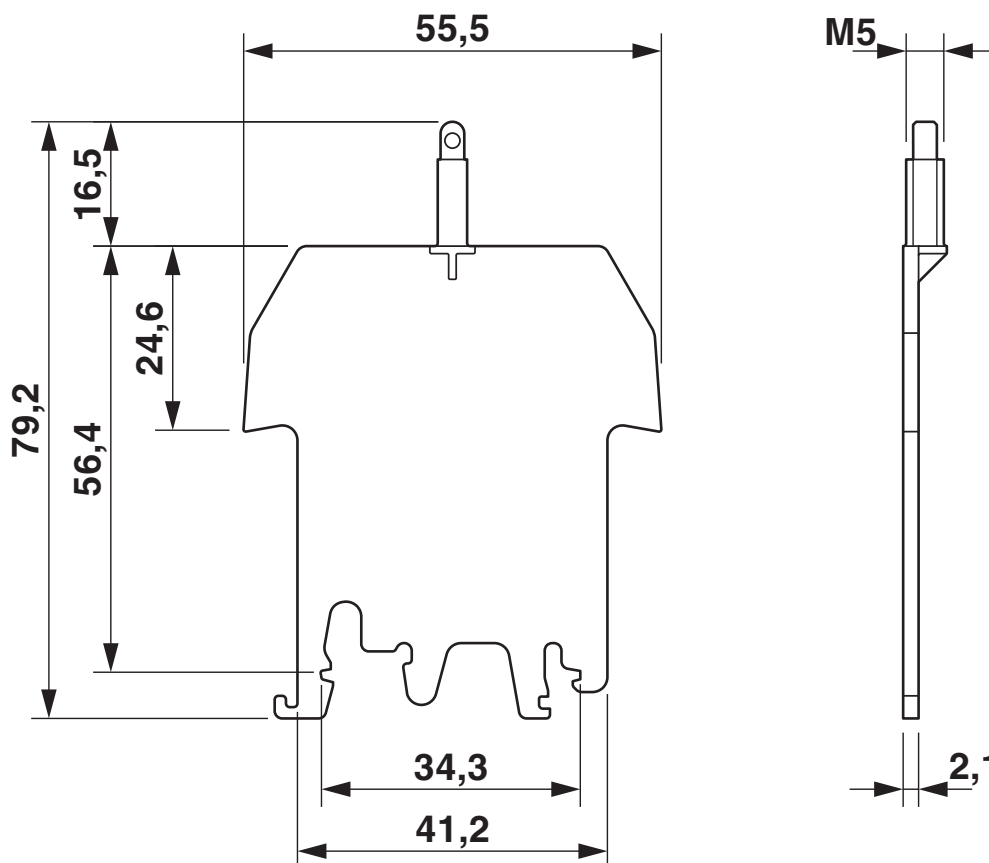
Dessin coté
