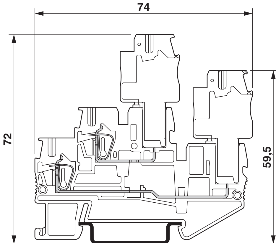
Maßzeichnung
