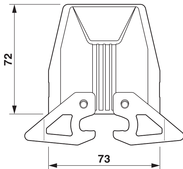
Dessin coté
