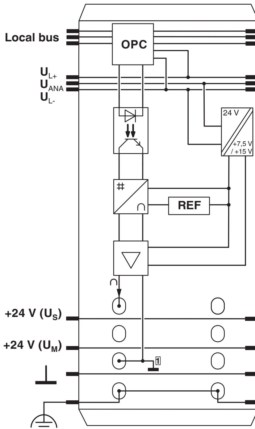
Schéma fonctionnel
