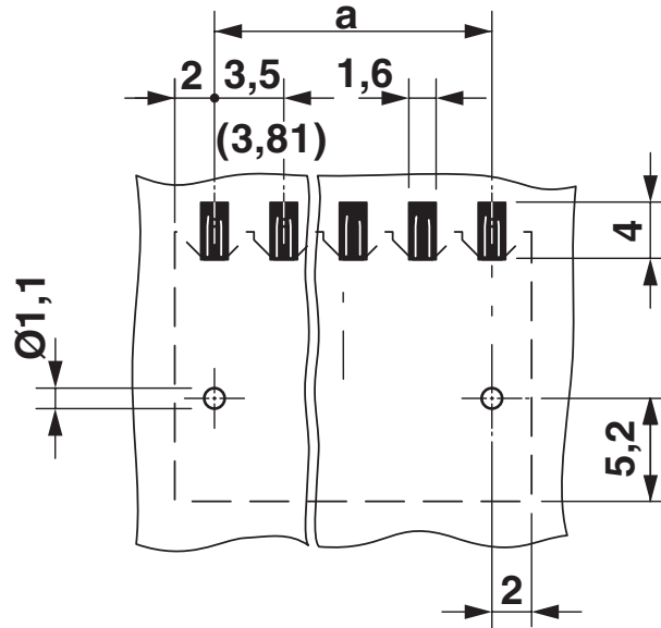
Bohrplan/Lötpadgeometrie
