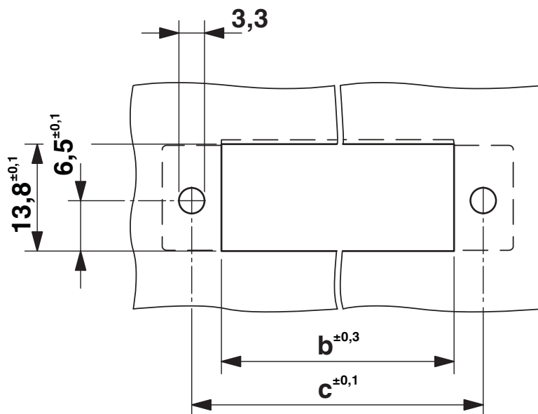
Maßzeichnung
