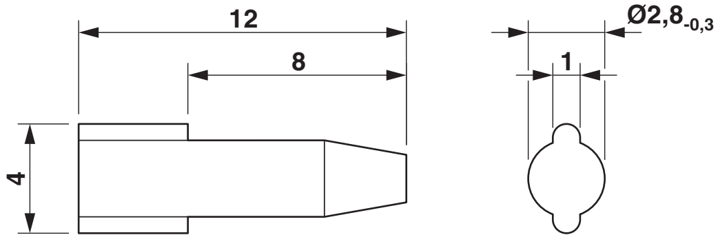
Maßzeichnung
