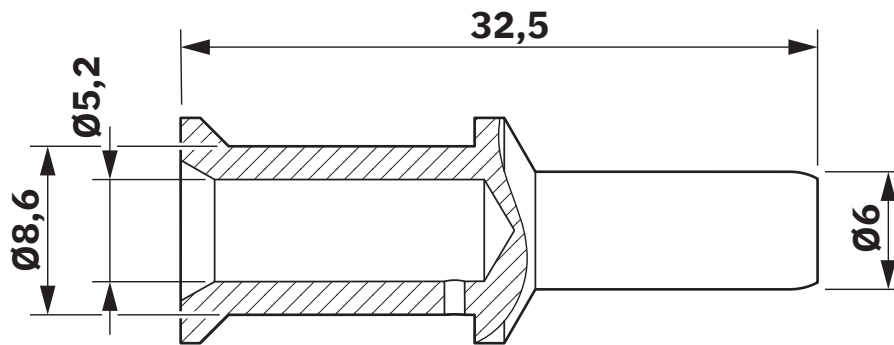
Maßzeichnung
