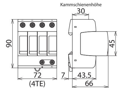
Maßbild DG M TT 320
