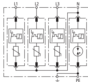
Prinzipialschaltbild DG M TT 320
