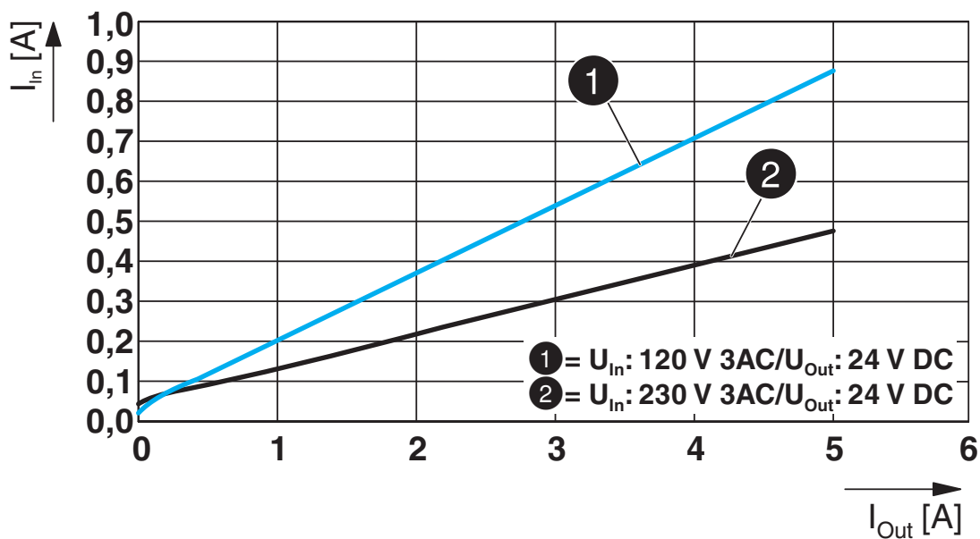
Eingangsstrom/Ausgangsstrom
