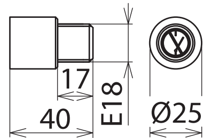
Maßbild SE E18
