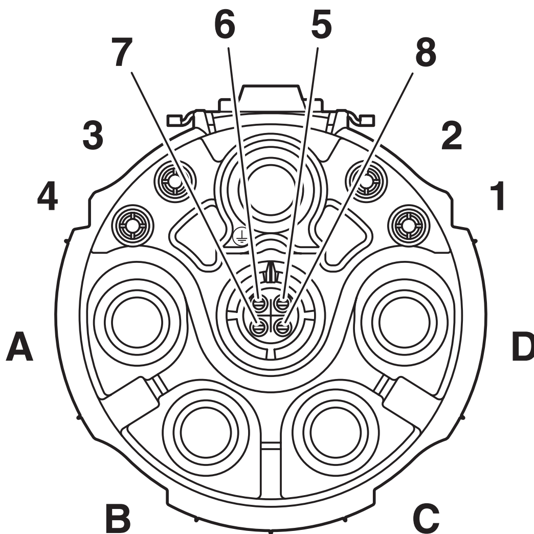
Dessin schématique
