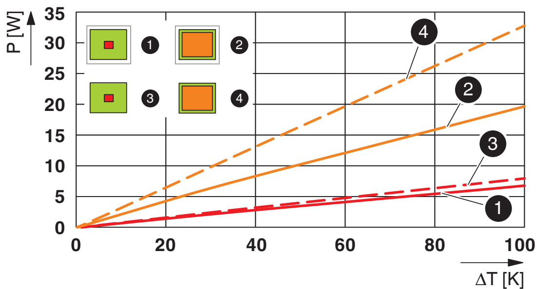
Diagrama de disipación de energía 0 K ... 100 K
