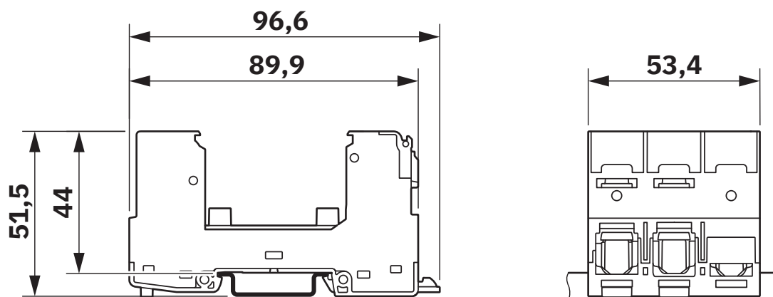
Maßzeichnung
