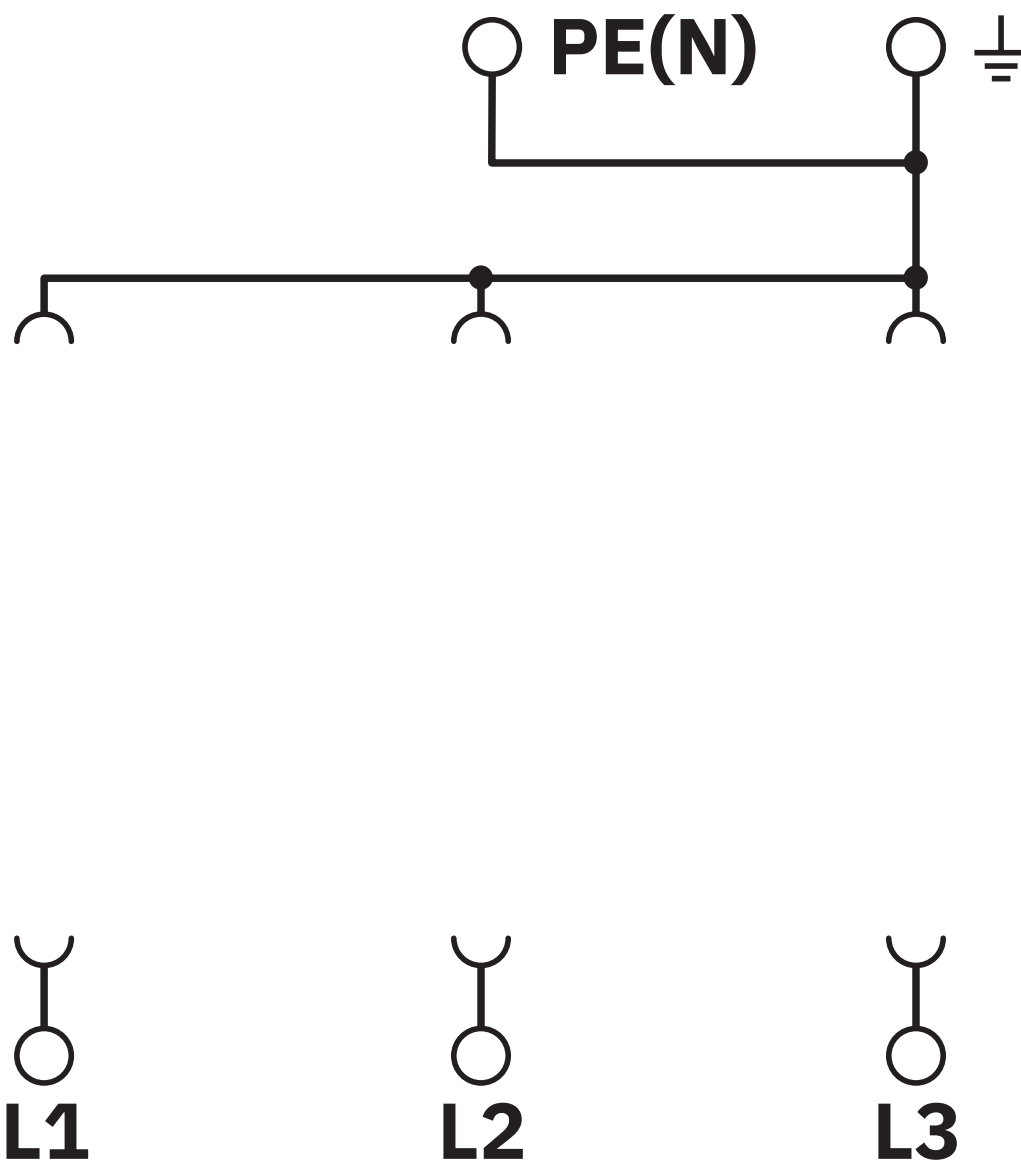
Diagrama eléctrico
