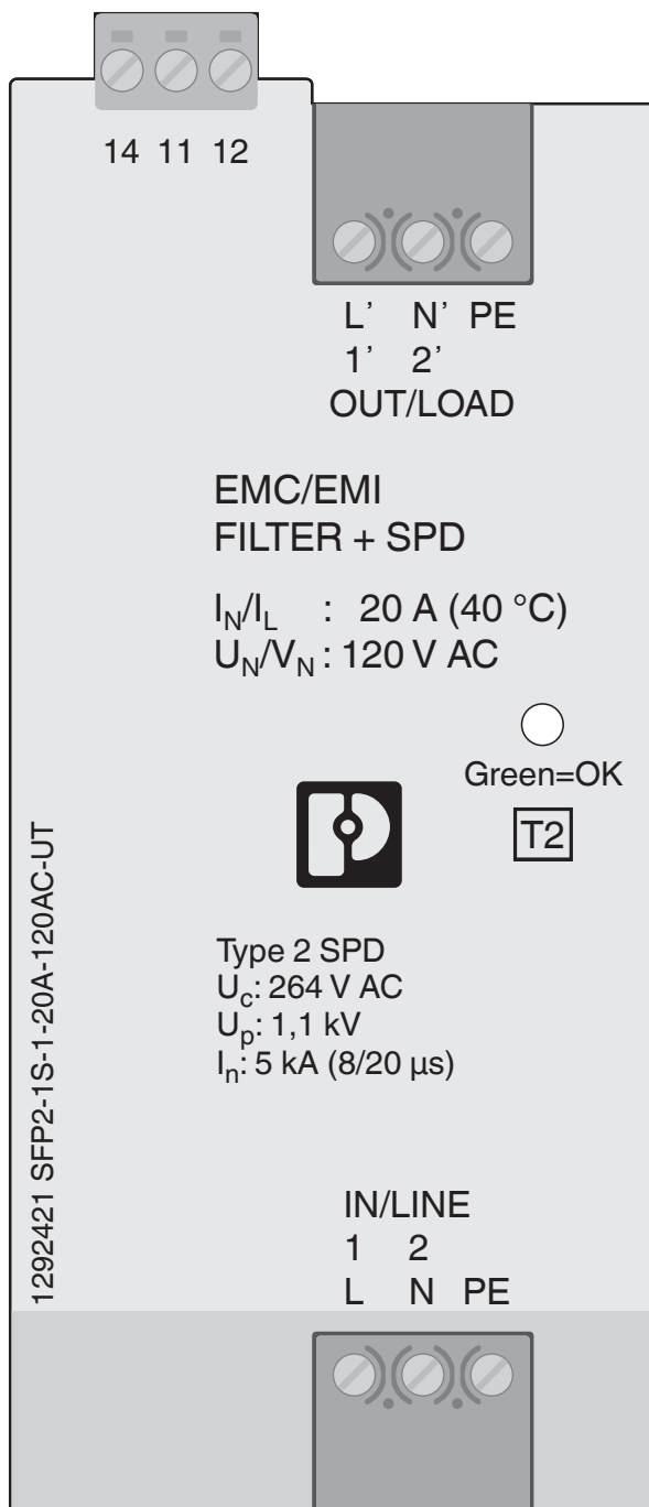
Produktzeichnung
