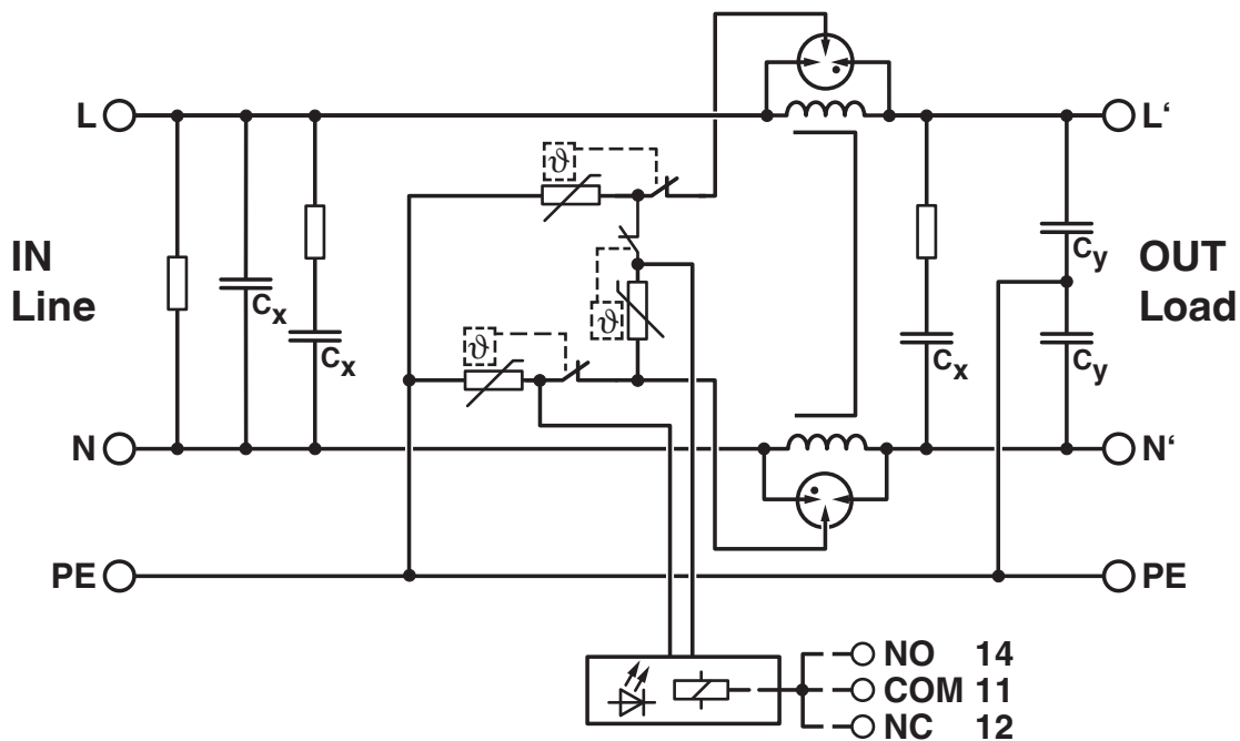
Diagrama eléctrico
