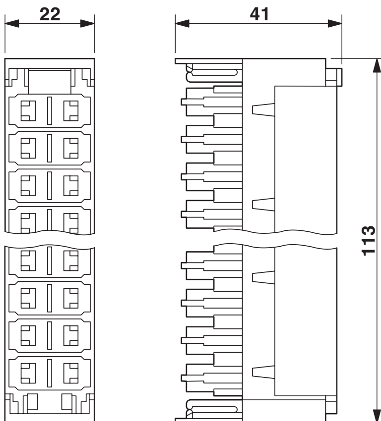
Dessin coté
