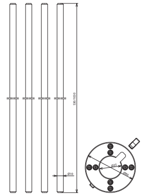
Maßbild BFRS D80 B35 4FSP 10 530 AL
