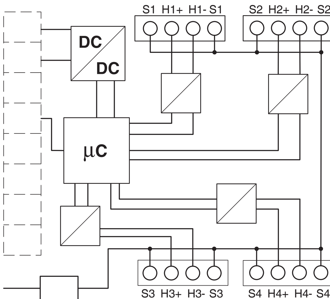
Schéma fonctionnel
