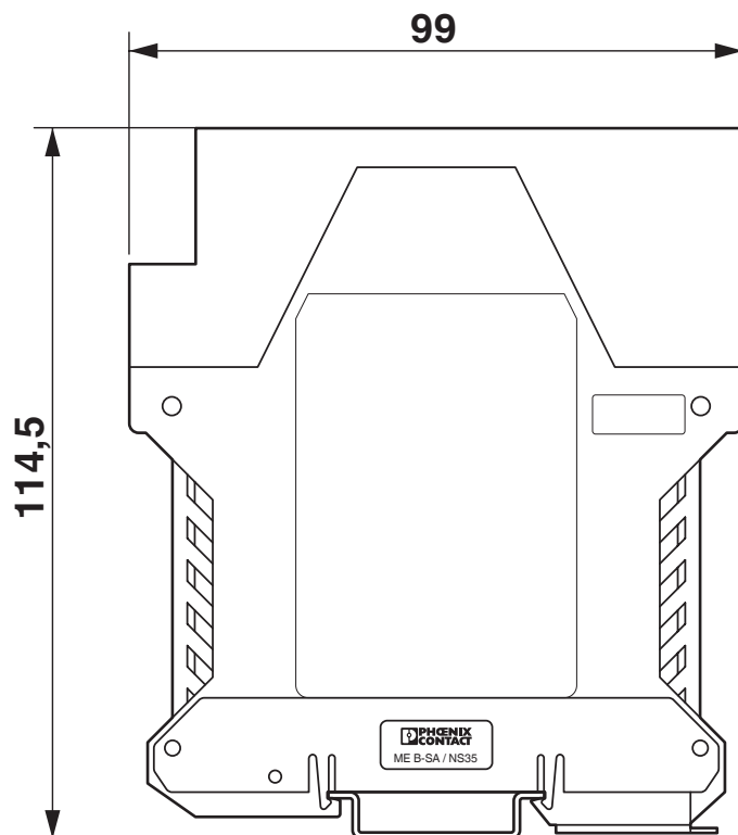
Dessin coté
