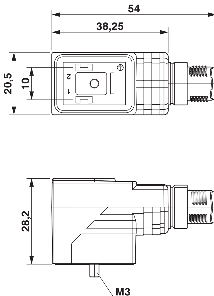
Dessin coté
