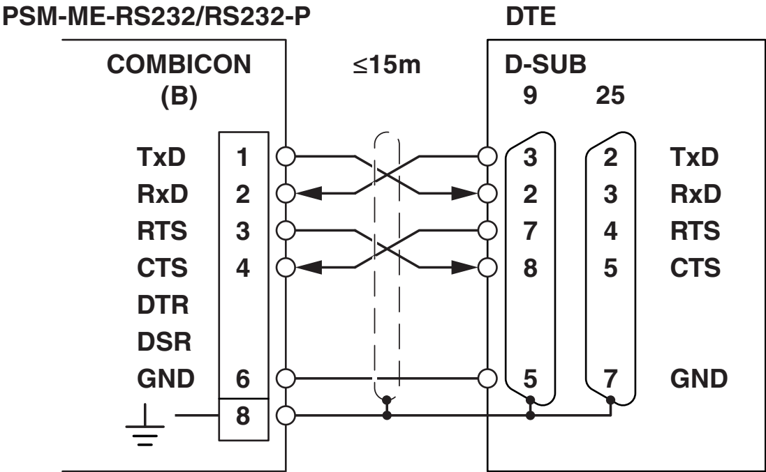
Conexión a un equipo DTE
