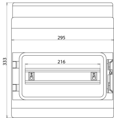
Dimensioni IGA 12 IP65
