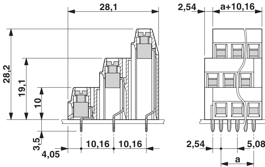
Maßzeichnung
