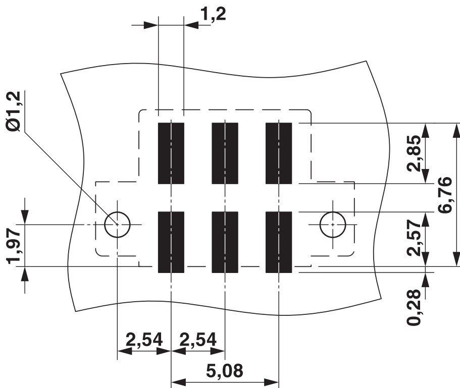
Esquema de taladros/geometría pads soldadura
