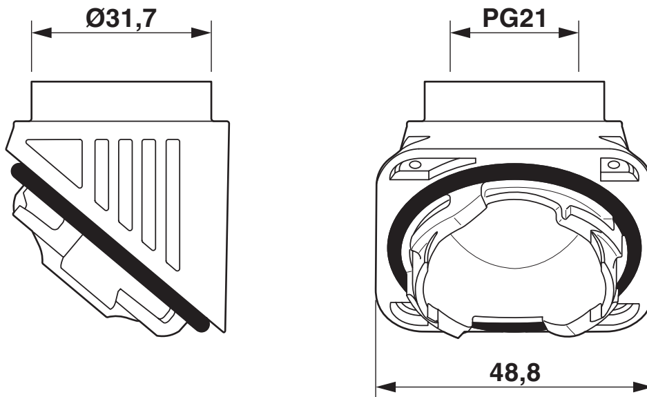
Maßzeichnung
