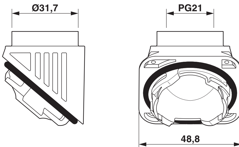
Dessin coté
