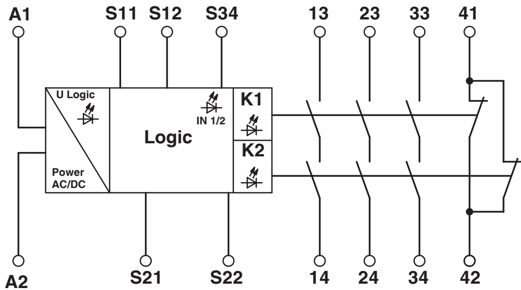
Diagrama eléctrico
