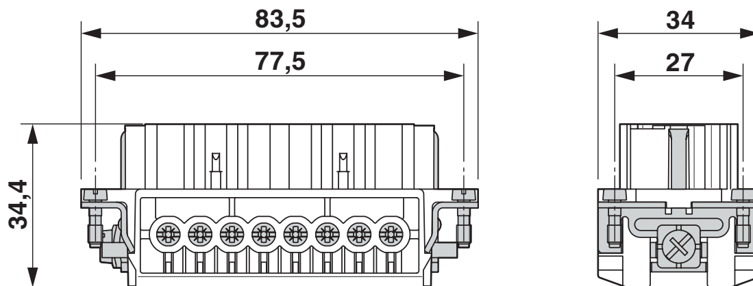
Dessin coté
