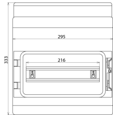
Dimensioni IGA 12 IP54
