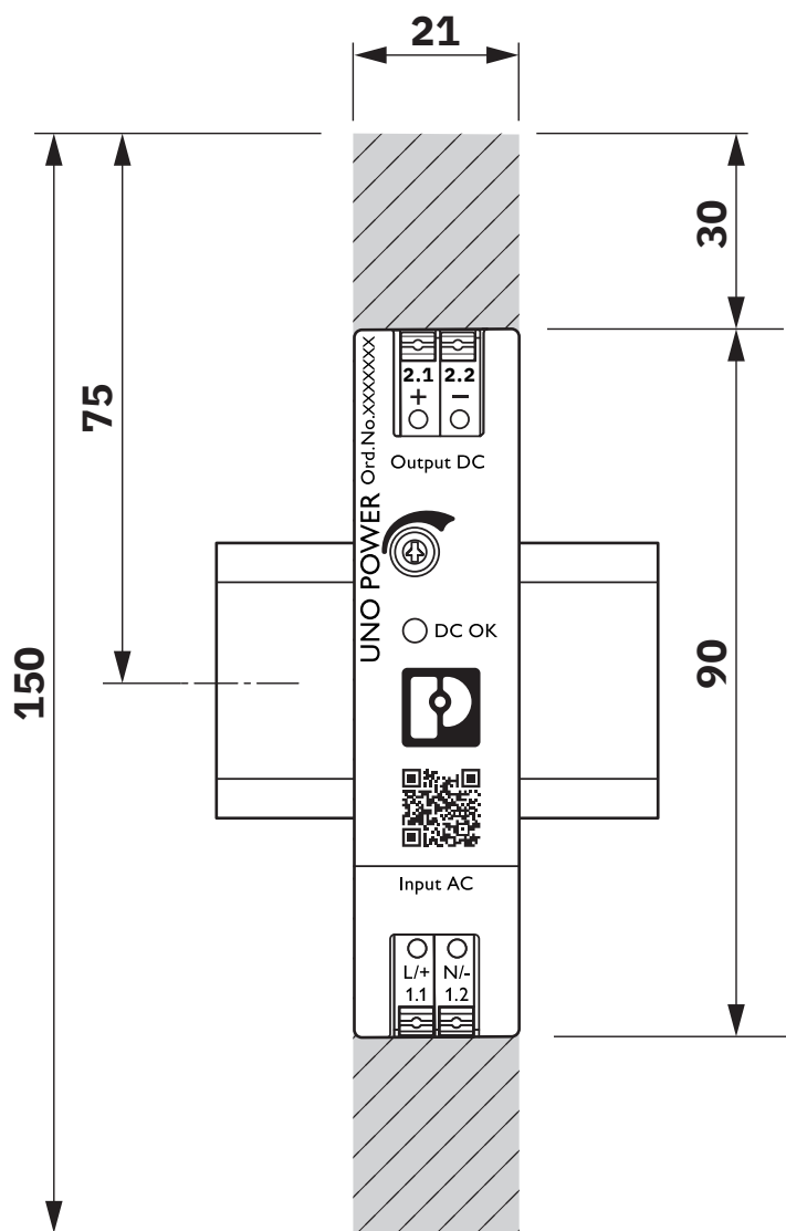
Maßzeichnung
