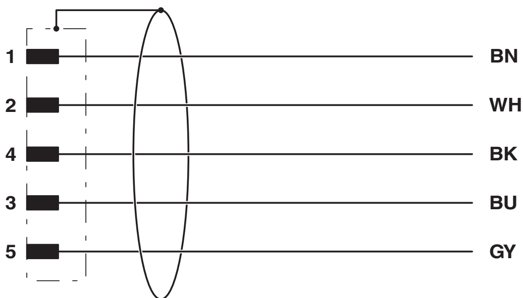
Diagrama eléctrico
