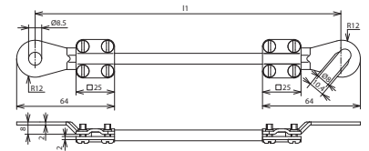
Maßbild EL10 L2.55M 1KSO 8.10 1KSG 8
