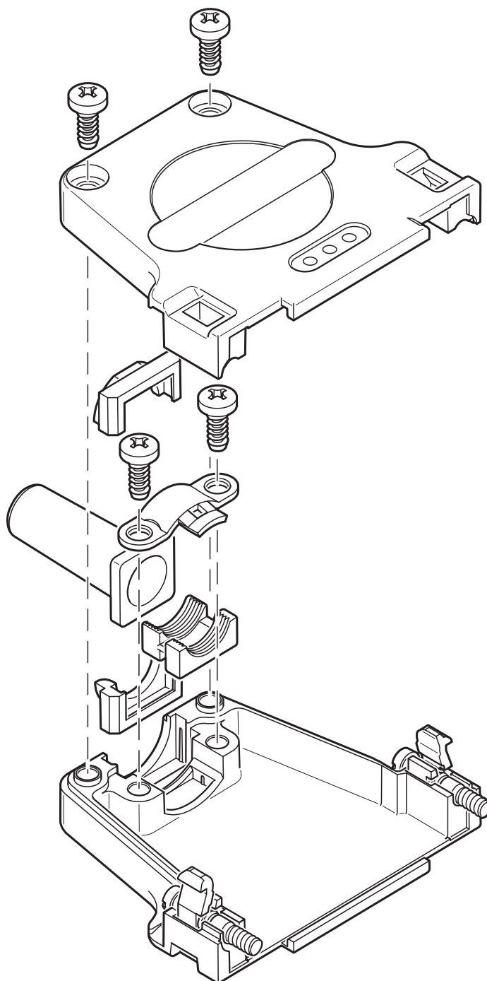
Plano esquemático
