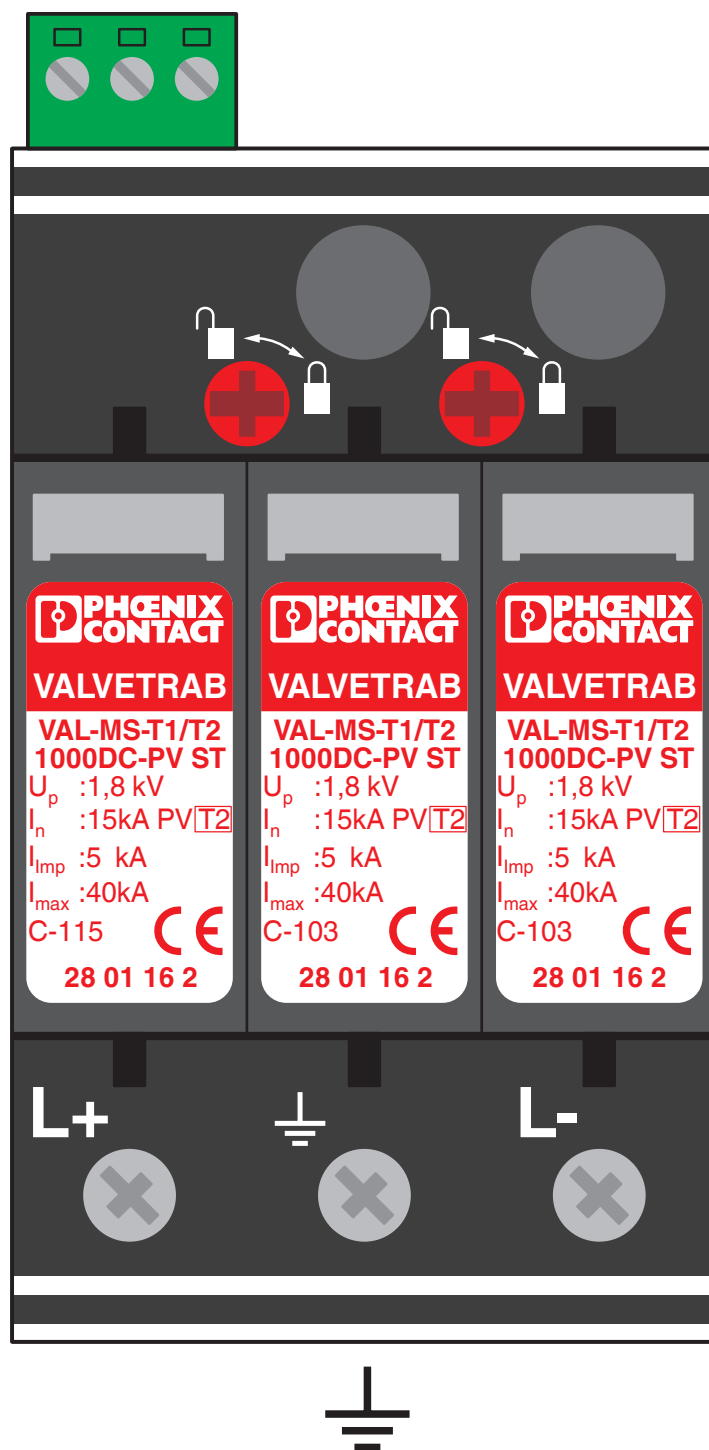
Dessin schématique
