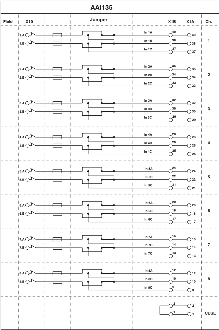
Schéma de connexion
