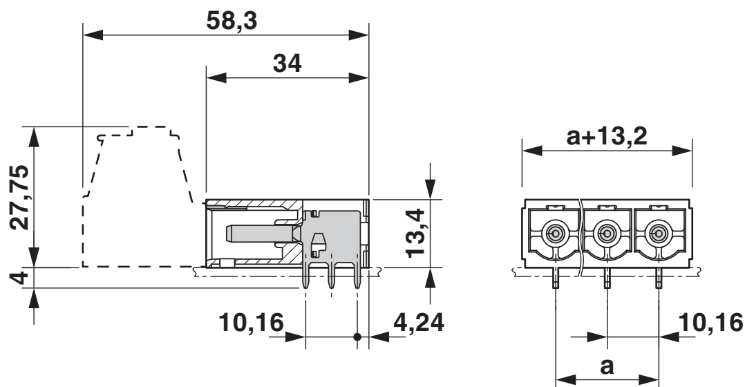
Dessin coté
