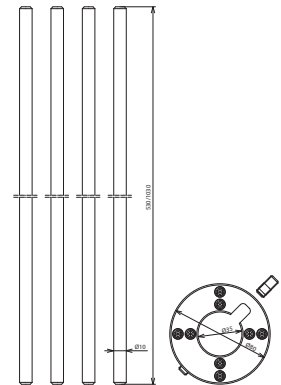
Maßbild BFRS D80 B35 4FSP 10 1030 V2A
