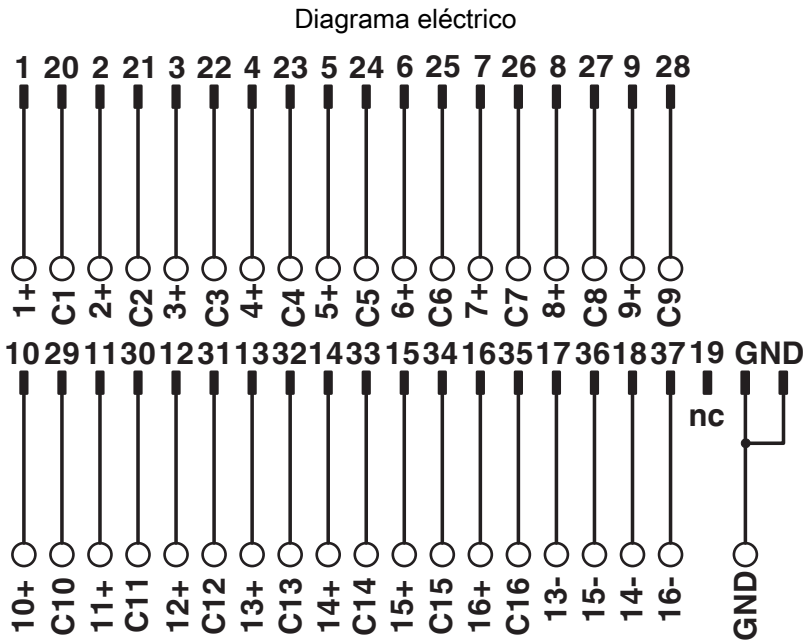
Esquema de conexiones VIP-3/.../D37SUB/M/HW/C300
