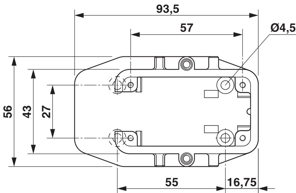
Maßzeichnung
