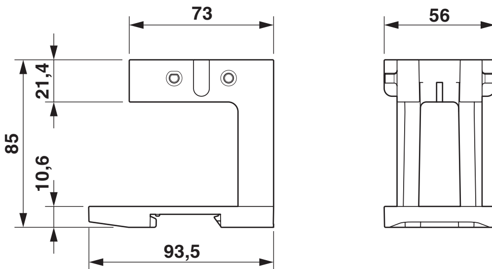
Maßzeichnung
