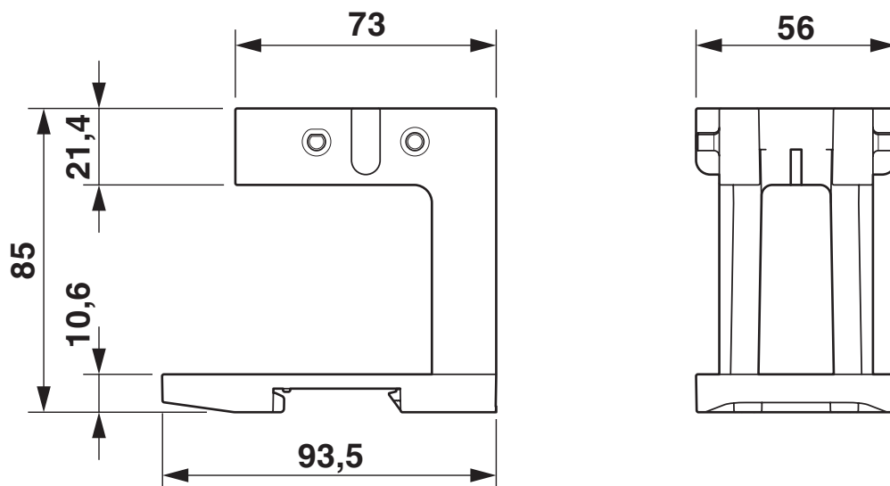
Dessin coté
