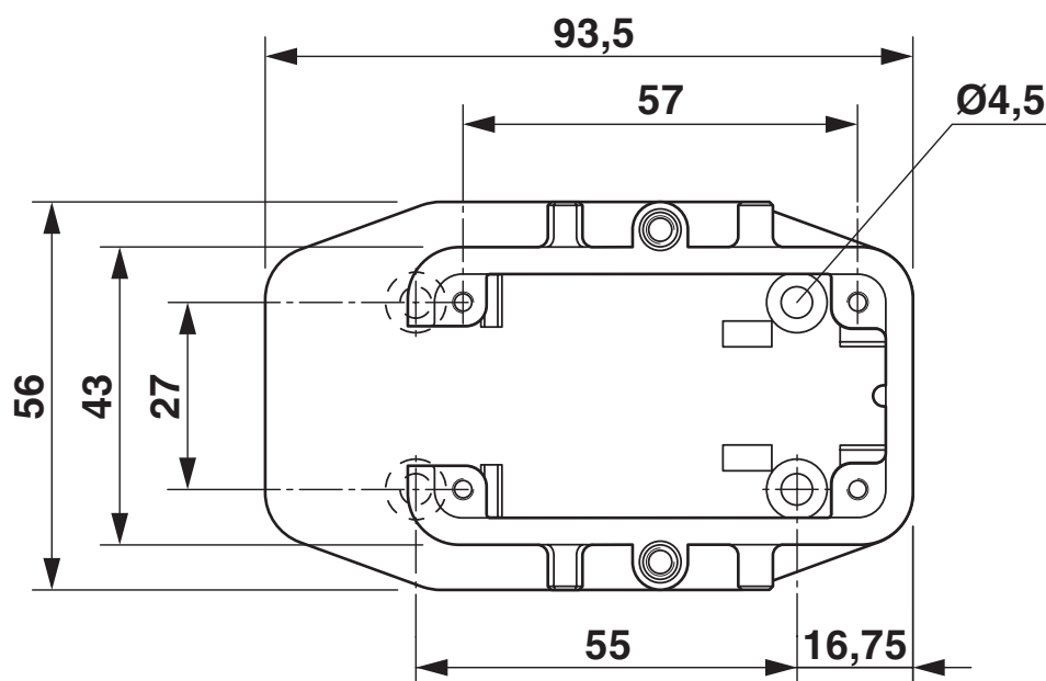
Dessin coté
